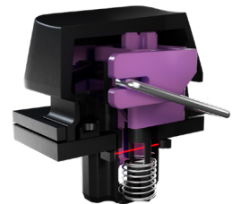
Razer オプト・メカニカル スイッチ構造
